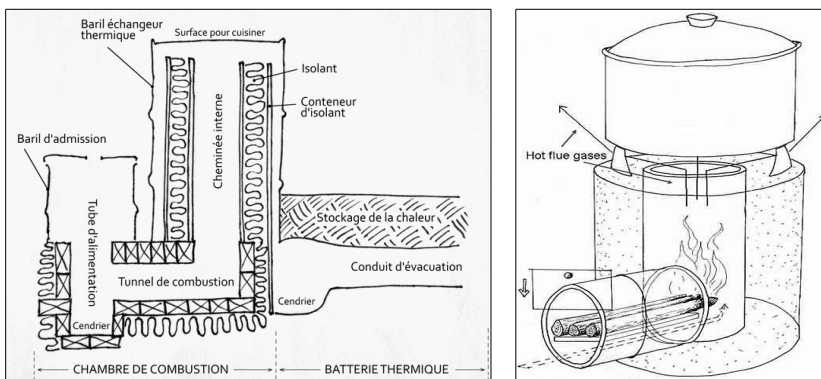
Rocket-Stove à gauche et cuiseur à bois à basse-consommation à droite.
