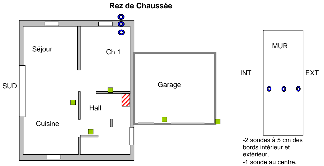
Figure 47 Schéma de principe des mesures (Maison paille)
